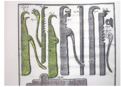
Abbildung 11 Konstruktionsplan „Pfaff-Zahngewerk“ 1756.
